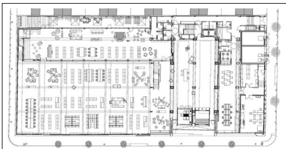
Figura 3. Biblioteca Montserrat Abelló i Soler: plànol de la planta baixa
